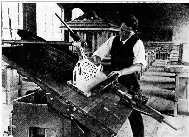
FIG. 161. RIPPING BEVELED EDGE STOCK.
